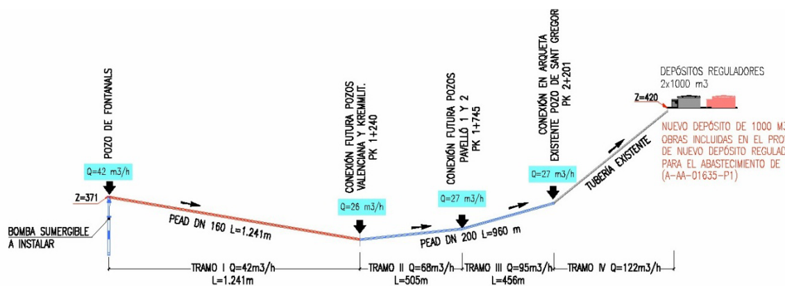
Esquema hidráulico de funcionamiento de las conducciones en alta de Falset
