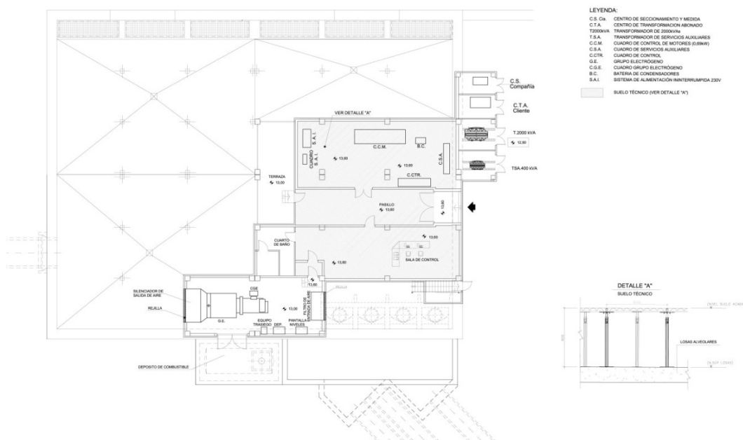
Planta general y planta interior del Tanque 2
